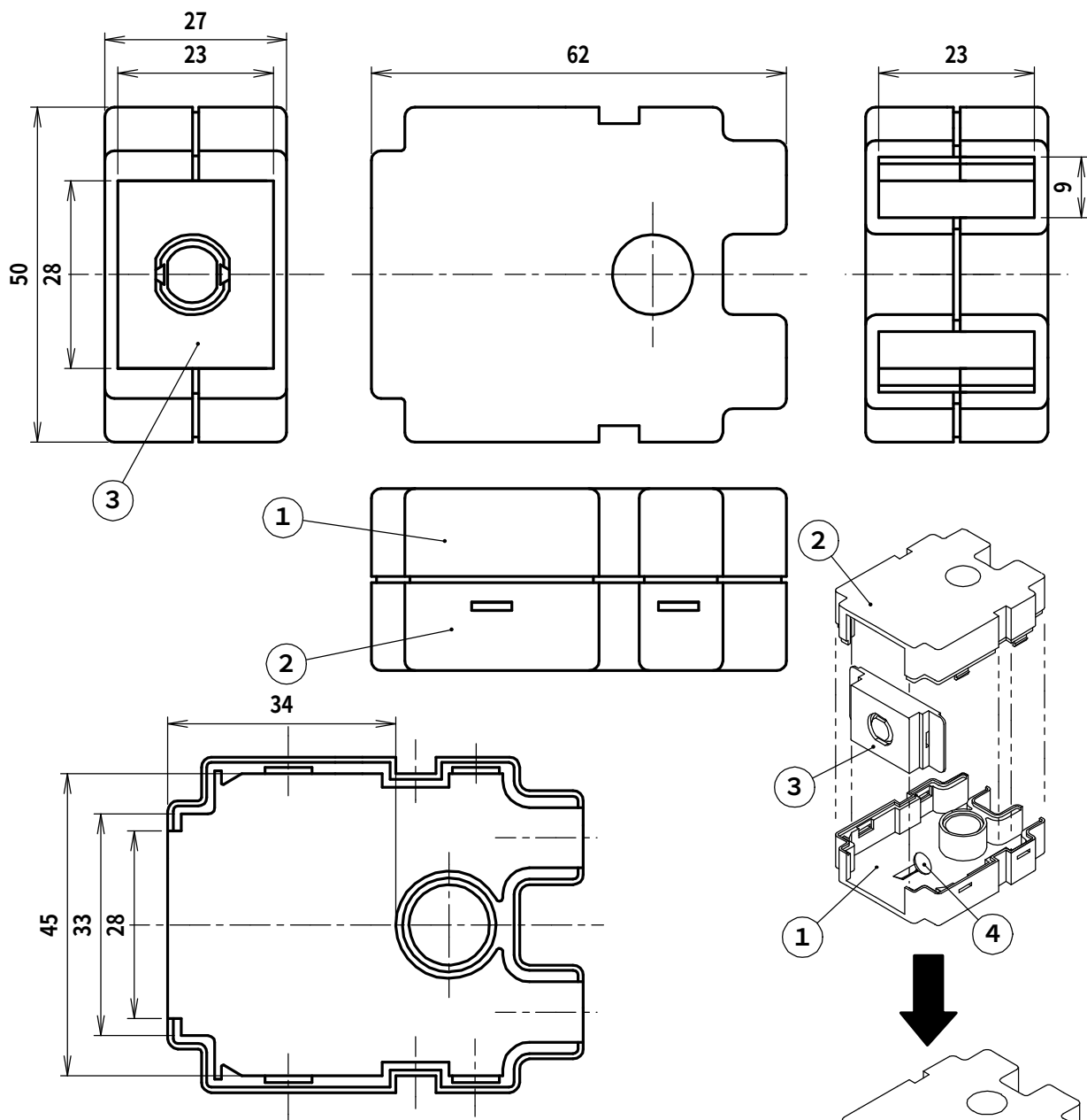
本体(メス)の内部寸法図(1/1)
